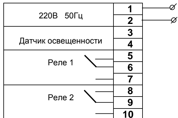
Схема подключения таймера реального времени ТРВ-02 «ТЕМП»
